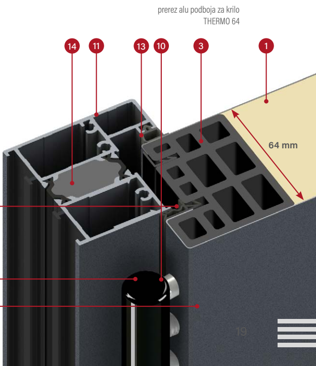
prerez jeklenega podboja za krilo THERMO 64
