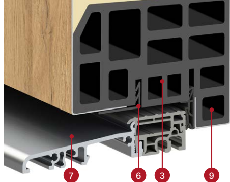
prerez krila THERMO HOT 88 s tesnilom in brez avtomatskega tesnila, alu prag
