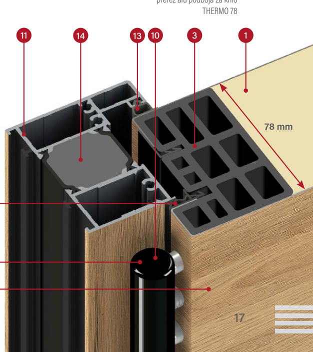
prerez alu podboja za krilo THERMO 78
