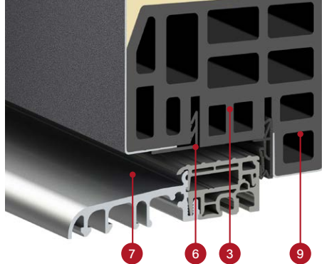
prezrez krila THERMO HOT 78 s tesnilom in brez avtomatskega tesnila, alu prag
