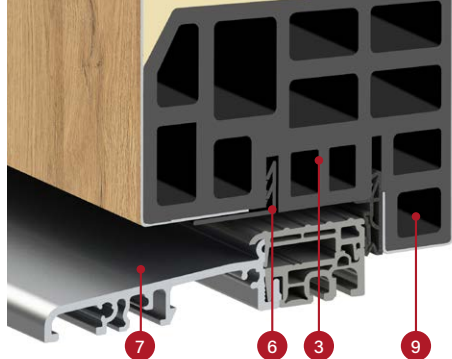
Secțiunea transversală a canatului THERMO HOT 88 cu garnitură și fără garnitură de etanșare podea, prag din aluminiu
