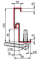
TOC DIN OȚEL DE COLȚ
