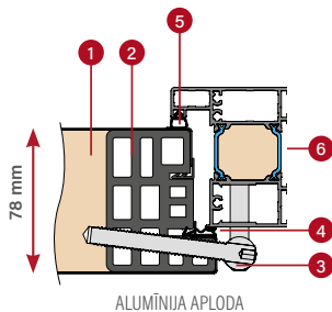
ALUMĪNIJA APLODA
