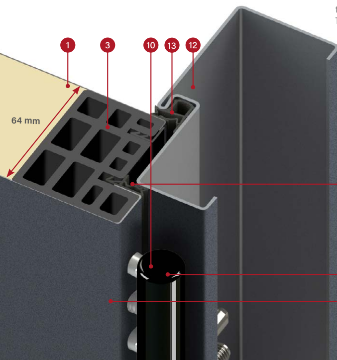
tērauda aploda durvju vērtnei THERMO 64 šķērsgriezums
