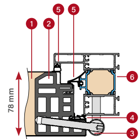
ALUMĪNIJA APLODA
