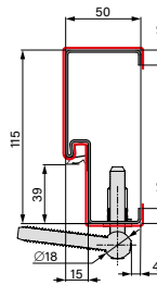
TĒRAUDA APLODA
