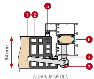
ALUMĪNIJA APLODA
