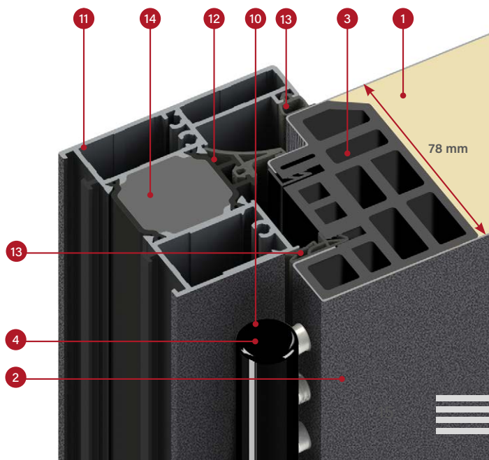
alumīnija aplodas durvju vērtnei THERMO HOT 78 šķērsgriezums
