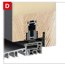
nolaižamā blīve 3)
