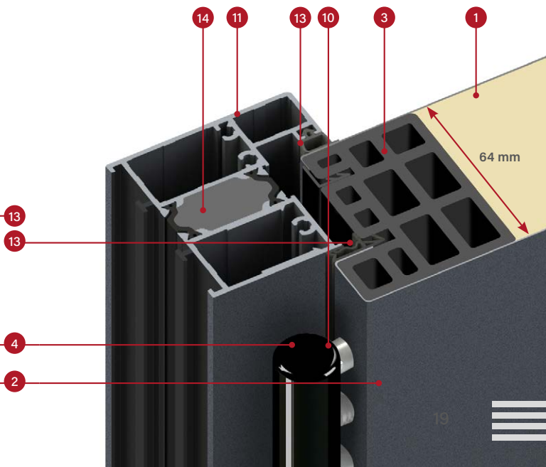
tērauda aploda durvju vērtnei THERMO 64 šķērsgriezums
