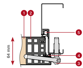
TĒRAUDA APLODA
