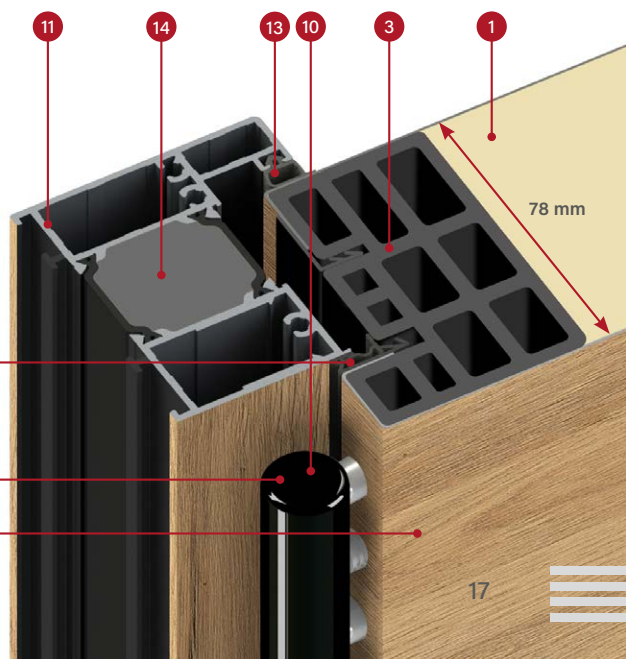
section du cadre en aluminium pour le vantail THERMO 78
