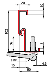
CADRE D'ANGLE EN ACIER
