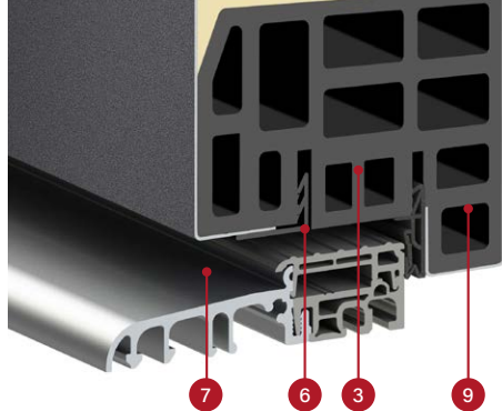
section du vantaill THERMO HOT 78 avec et sans joint de bas de porte, seuil en aluminium
