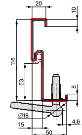
CADRE D'ANGLE EN ACIER
