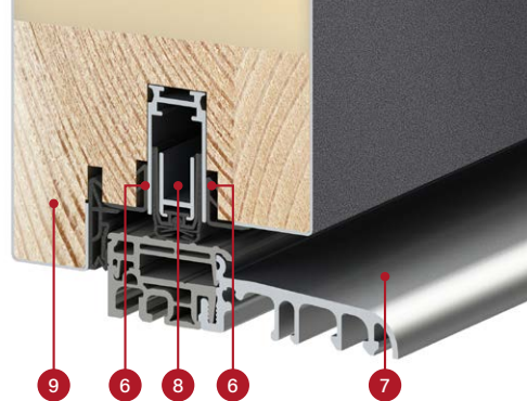
section du vantaill THERMO HOT 78 avec et sans joint de bas de porte, seuil en aluminium
