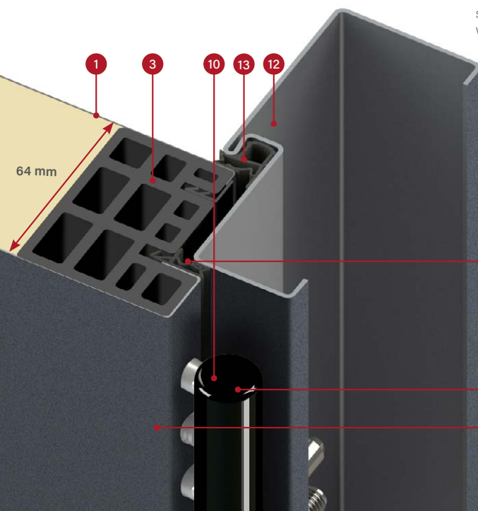
section du cadre en acier pour le vantail THERMO 64
