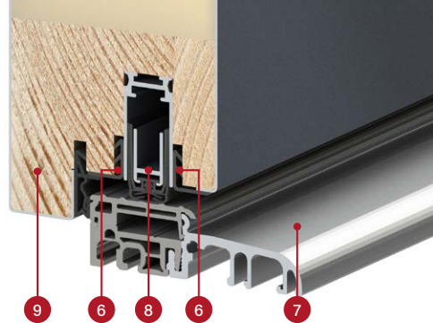
section du vantail THERMO 64 avec et sans joint de bas de porte, seuil en aluminium
