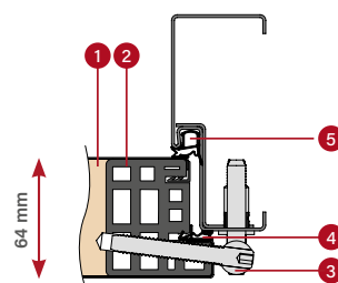
CADRE EN ACIER
