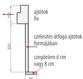
ajtótok bővítése
