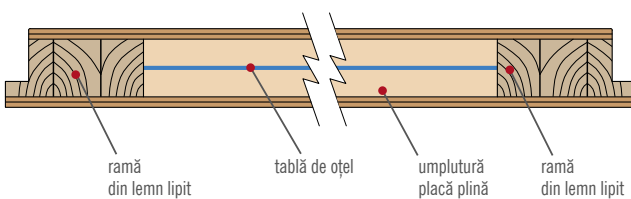
PRAG DIN TABLĂ INOXIDABILĂ
