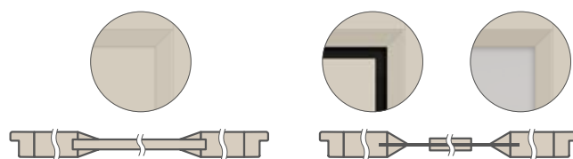
WERBENA 1, 2, 3 Profil înclinat subțire lângă panoul de 16 mm
