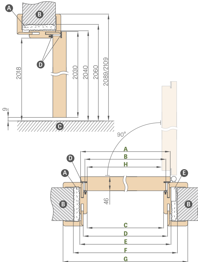
SCHEMĂ TOC REGLABIL HERSE SET
