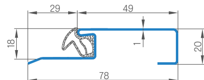
PRAG DIN TABLĂ INOXIDABILĂ
