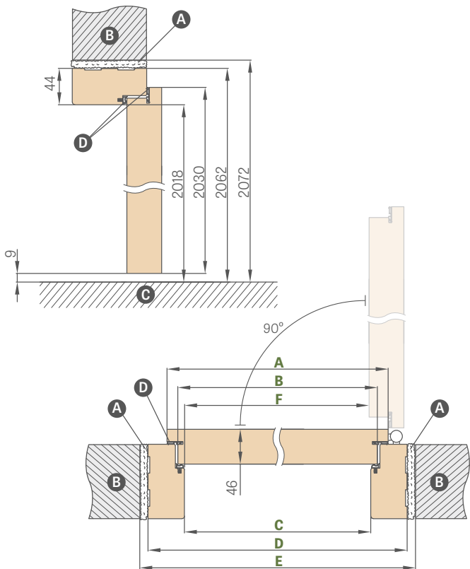
SCHEMĂ TOC FIX HERSE SET
