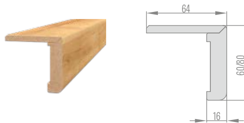
COLȚAR CU LIMBĂ PRELUNGITĂ PENTRU TOC REGLABIL
