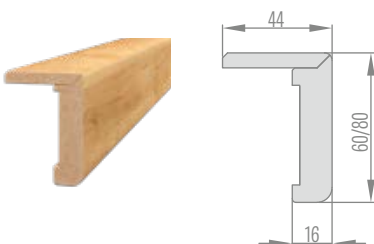
СТАНДАРДЕН АГОЛ ЗА ПРИЛАГОДЛИВА РАМКА НА ВРАТА
