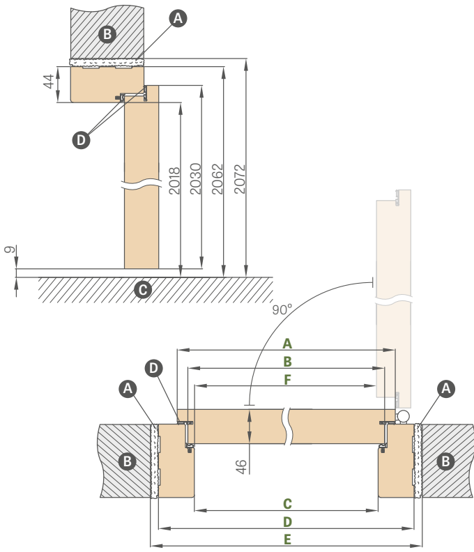
ДИЈАГРАМ НА ФИКСИРАНА РАМКА НА ВРАТАТА ОД HERSE SET
