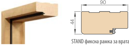
STAND фиксна рамка за врата
