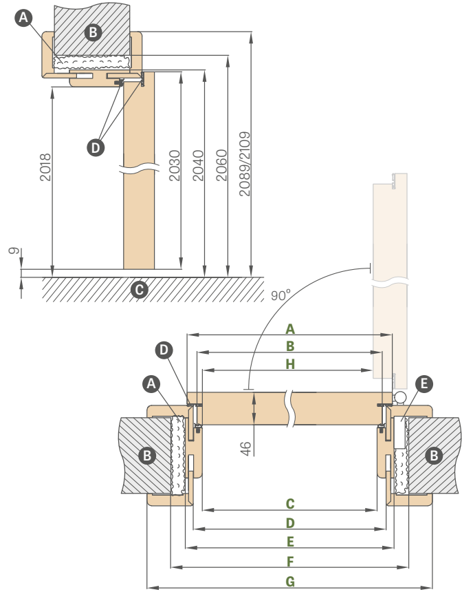
ДИЈАГРАМ НА ПРИЛАГОДЛИВАТА РАМКА НА ВРАТАТА ОД HERSE SET
