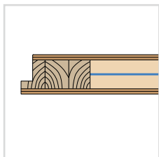
VANTAIL de 46 mm renforcée par une tôle d'acier
