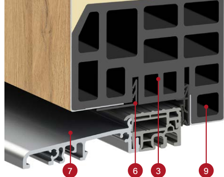
przekrój skrzydła THERMO HOT 88 z uszczelką i bez uszczelki opadającej, próg aluminiowy
