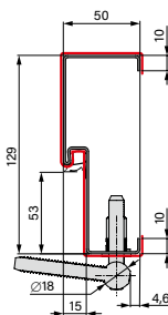
OŚCIEŻNICA STALOWA
