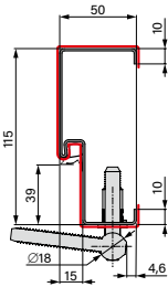
OŚCIEŻNICA STALOWA
