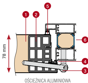
OŚCIEŻNICA ALUMINIOWA
