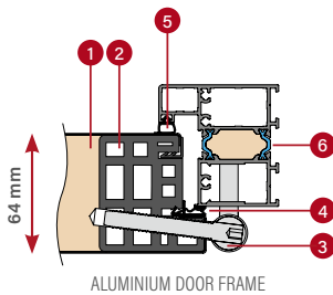
ALUMINIUM DOOR FRAME
