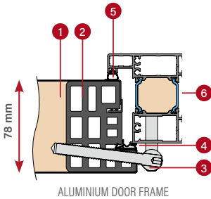
ALUMINIUM DOOR FRAME
