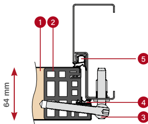
STEEL DOOR FRAME
