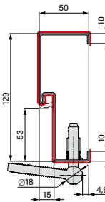
STEEL DOOR FRAME
