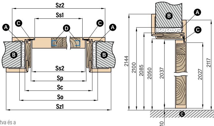
A – puhhab B – fal C – tömítés D – acél U-profil
