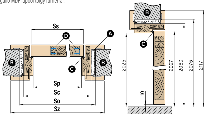
A – puhhab B – fal C – tömítés D – acél U-profil
