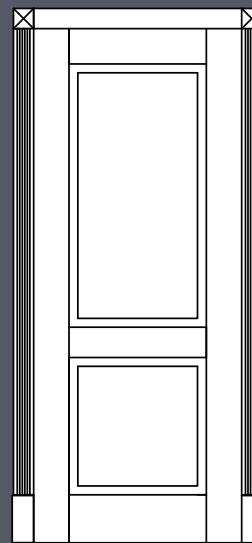
ДЕКОРАТИВНІ ОПАСКИ OP-4 ■ верхні конверти ■ нижні стовпчики ■ доплата
