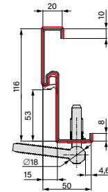
ДВЕРНА КОРОБКА СТАЛЕВА КУТОВА
