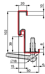
ДВЕРНА КОРОБКА СТАЛЕВА КУТОВА
