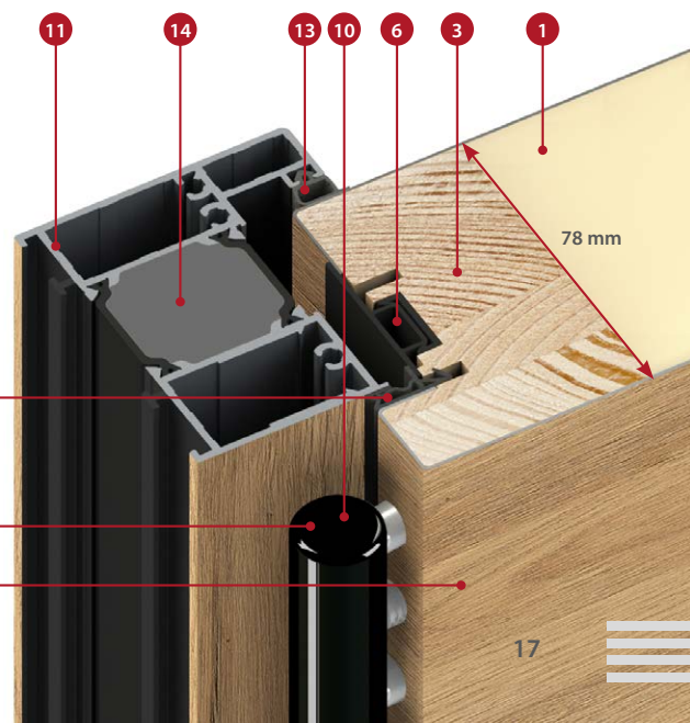
поперечний переріз алюмінієву дверної коробки для стулки THERMO 78
