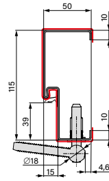
ДВЕРНА КОРОБКА СТАЛЕВА
