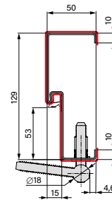
ДВЕРНА КОРОБКА СТАЛЕВА
