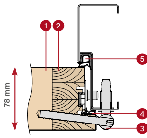
TĒRAUDA APLODA
