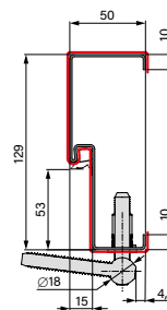
TĒRAUDA APLODA
