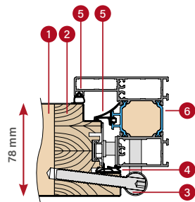
ALUMĪNIJA APLODA
