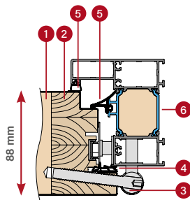
ALUMĪNIJA APLODA
