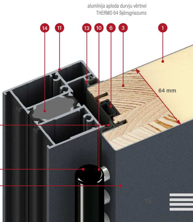
tērauda aploda durvju vērtnei THERMO 64 šķērsgriezums
