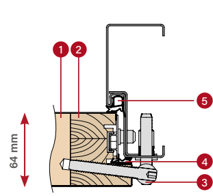
TĒRAUDA APLODA
