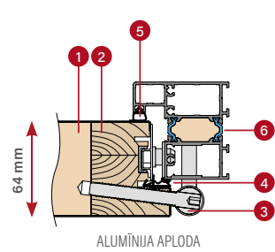
ALUMĪNIJA APLODA
