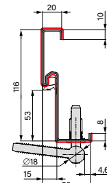
ROHOVÁ OCELOVÁ ZÁRUBEŇ
