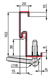
ЪГЛОВА СТОМАНЕНА КАСА
