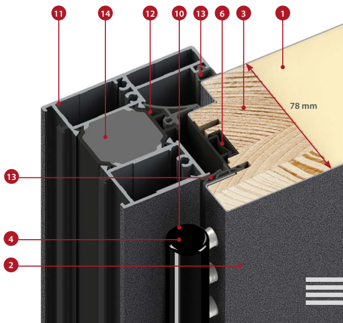
напречно сечение на алуминиева каса за крило THERMO HOT 78
