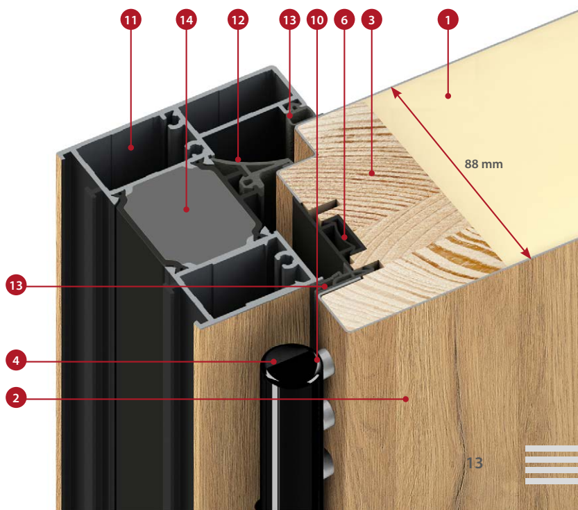
напречно сечение на алуминиева каса за крило THERMO HOT 88
