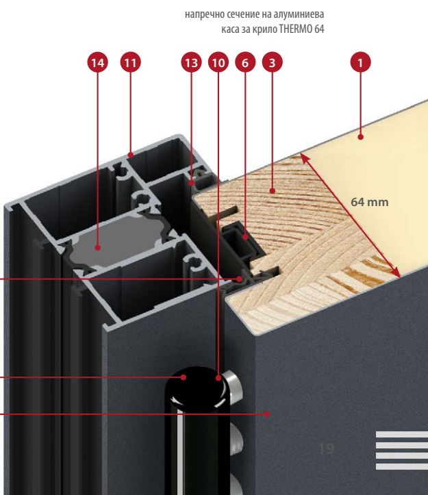
напречно сечение на стоманена каса за крило THERMO 64
