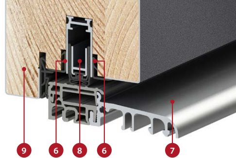
напречно сечение на крило THERMO HOT 78 със и без падащо уплътнение, алуминиев праг
