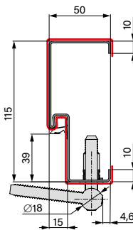
OCELOVÁ ZÁRUBEŇ
