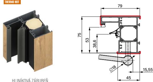
HLINÍKOVÁ ZÁRUBEŇ
