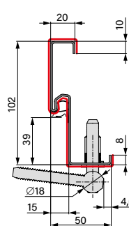
ROHOVÁ OCELOVÁ ZÁRUBEŇ
