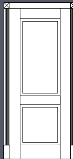
OZDOBNÉ OBLOŽKY OP-4 ■ horné obálky ■ spodné stĺpiky ■ príplatok
