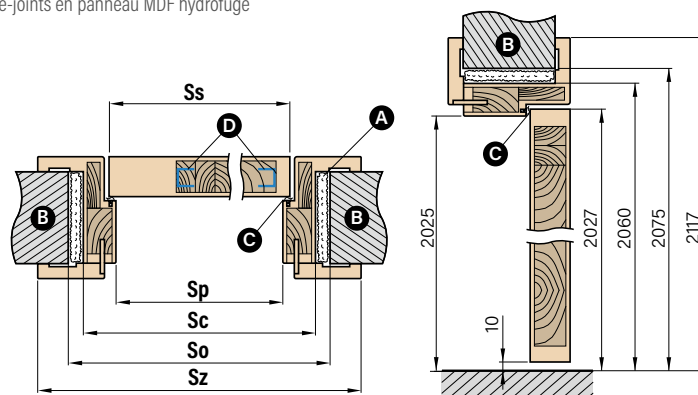
A - mousse de montage B - mur C - joint d'étanchéité D - profil en U en acier
