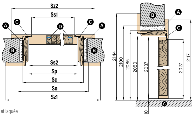
A - mousse de montage B - mur C - joint d'étanchéité D - profil en U en acier
