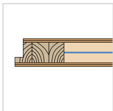
KRÍDLO 46 mm zosilnené ocelovým plechom
