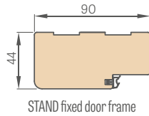
STAND fixed door frame
