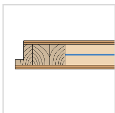
VANTAIL 46 mm renforcé de tôle d'acier
