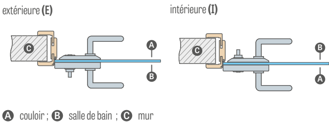
Panneau de remplissage spécial HALSPAN : 44 mm [EI30] / 54 mm [EI60]
