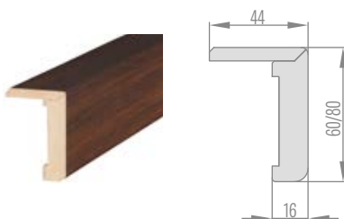
CORNIÈRE STANDARD POUR DORMANT RÉGLABLE
