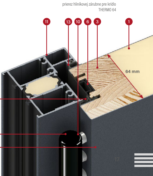
prierez ocelevej zárubne pre krídlo THERMO 64
