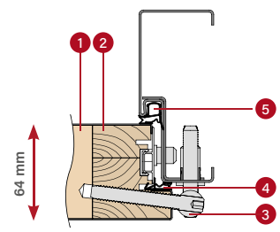
OCEĽOVÁ ZÁRUBŇA
