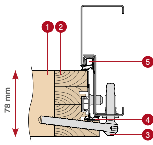
OCEĽOVÁ ZÁRUBŇA
