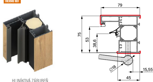
HLINÍKOVÁ ZÁRUBEŇ
