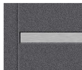
Oboustranné prolisy o šířce 25 mm s intarzií s povrchovou úpravou INOX nebo lakovanou načerno. Intarzií je možné montovat jednostranně nebo oboustranně. Vkládá se do prolisu a je v jedné rovině s křídlem (STAMP) nebo nalepená na ploché dveřní křídlo (LABEL).
