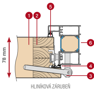
HLINÍKOVÁ ZÁRUBEŇ
