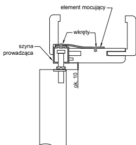
RYSunEK 3. Łączenie prowadnicy ze wzmocnieniem – przekrój poprzeczny
