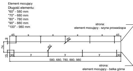
RYSunEK 3. Łączenie prowadnicy ze wzmocnieniem – przekrój poprzeczny
