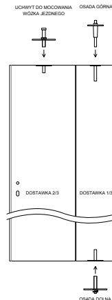
RYSunEK 4. Drzwi składane - dostawki
