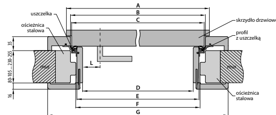
Schemat ościeżnicy nakładkowej – rzut z góry
