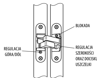
1BP ZAWIAS UKRYTY
